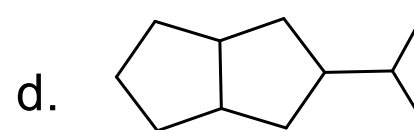
3-isopropilbiciclo[3.3.0]ottano
