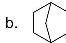
biciclo[2.2.1]eptano
