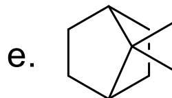
7,7-dimetilbiciclo[2.2.1]eptano
