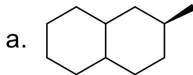
(3S)-3-metilbiciclo[4.4.0]decano
