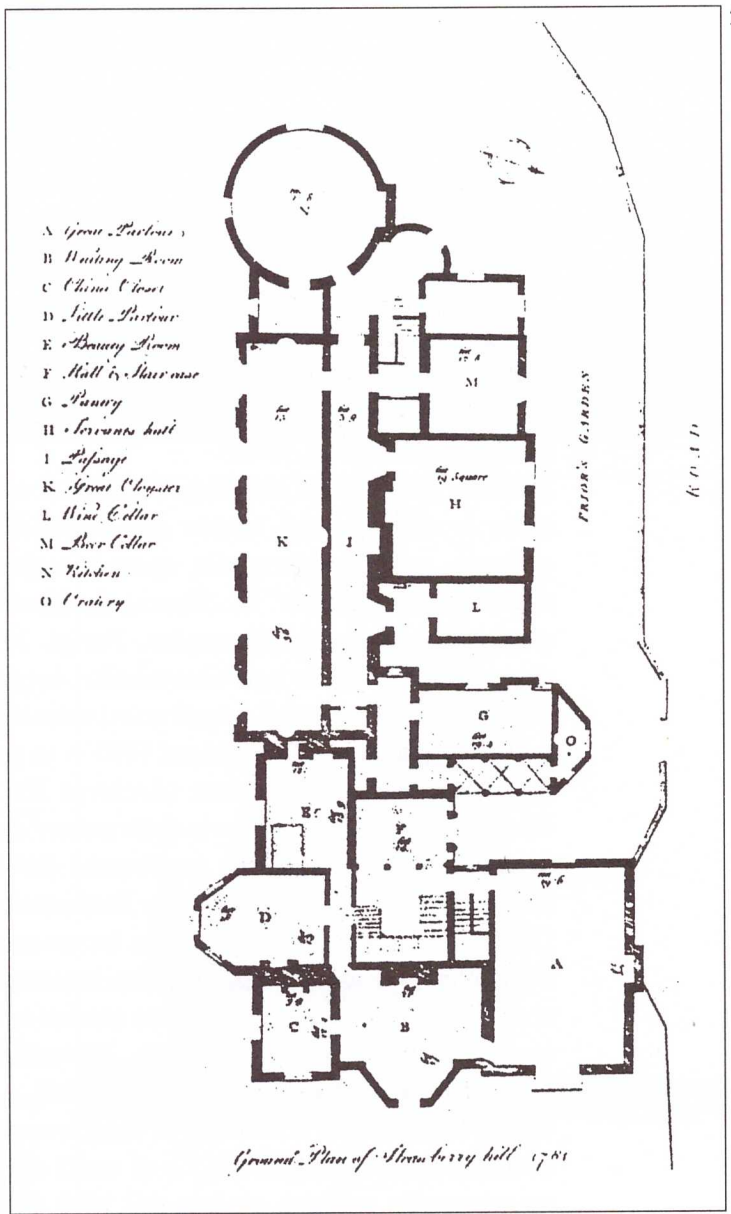
FIGURA 2 • Strawberry Hill (dintorni di Twickenham, Gran Bretagna) pianta di progetto per il piano terreno, 1781. Richard Bentley è probabilmente colui che ha caratterizzato Strawberry Hill nella sua originale fisionomia gotico-rococò voluta da Walpole. Egli è stato forse il primo fautore del gotico ad insistere sulla necessità di copiare opere del passato. Peraltro, benché le ricerche archeologiche di Walpole costituiscano una novità nello sviluppo del revival, egli se ne serve secondo il gusto del suo tempo, allo stesso modo di Bentley, un uomo dall'inventiva sbrigliata, che, al pari del suo committente è attirato specialmente dagli aspetti leggeri e graziosi del gotico come mostra anche l'articolazione planimetrica dell'edificio (da Walpole, 1990).
