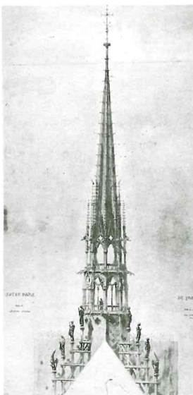
FIGURE 10-11 • Parigi. Notre-Dame, progetto della guglia centrale (29 ottobre 1857, Centre de Recherches des Monuments Historiques, Parigi) e dettaglio all'incrocio del transetto. Con la rivoluzione del 1789 la cattedrale subisce gravi danni e solo dopo il 1815 si può pensare al suo restauro che si comincia a concretizzare nel 1845 per concludersi diciannove anni dopo. Tra i lavori è prevista anche la ricostruzione della guglia centrale che sviluppa novantasei metri di altezza. Essa è posta all'incrocio delle coperture delle navate e del transetto; un punto sottolineato anche dalle figure scultoree che Viollet-le-Duc scaglionava lungo le linee d'intersezione (da AA.VV., 1981a).
