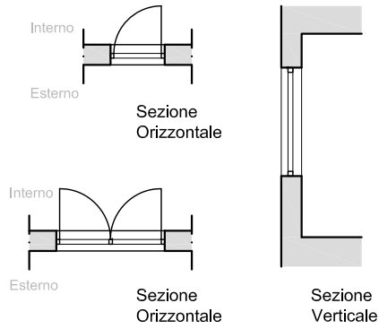
Finestra Scala 1:100
