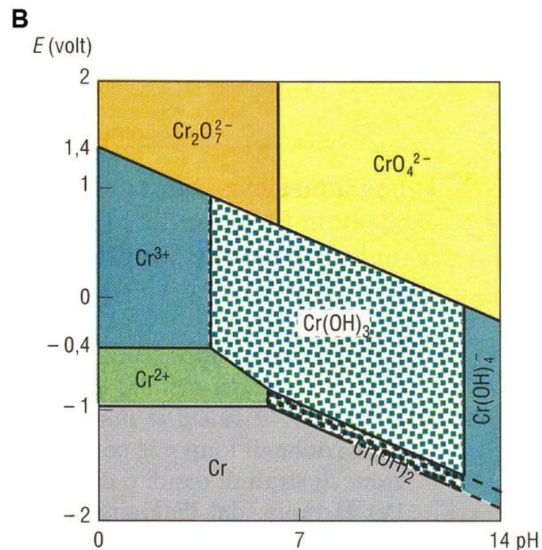
Potenziali redox in funzione del pH: ferro (A) e cromo (B)
