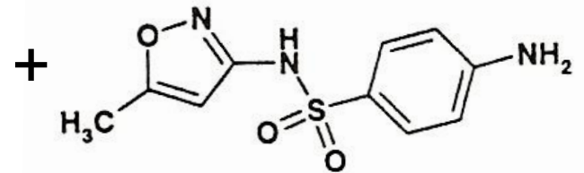
Sulfamethoxazole
