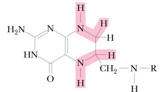
Tetraidrofolato
