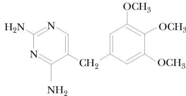
Trimetoprim
