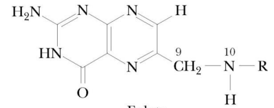
Folato
