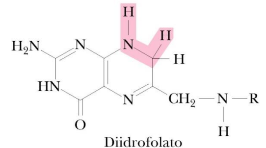
Diidrofolato
