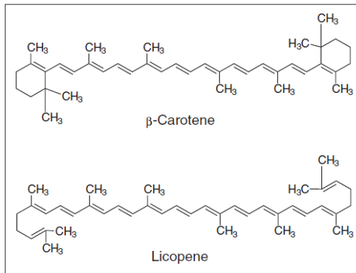
Figura 6.14 Struttura del \beta -carotene e del licopene (caroten).
