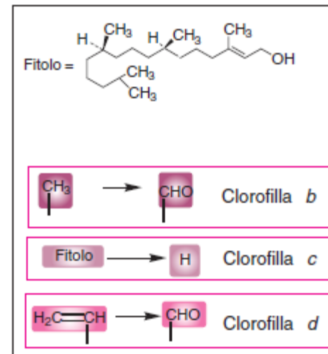
Figura 6.12 Struttura delle clorofille.
