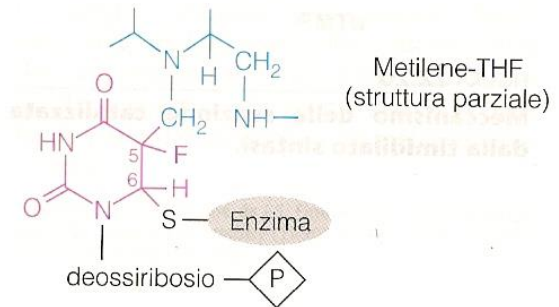
Complesso tra dUMP legato all'enzima e il 5,10-metilene-THF
