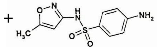
Sulfamethoxazole
