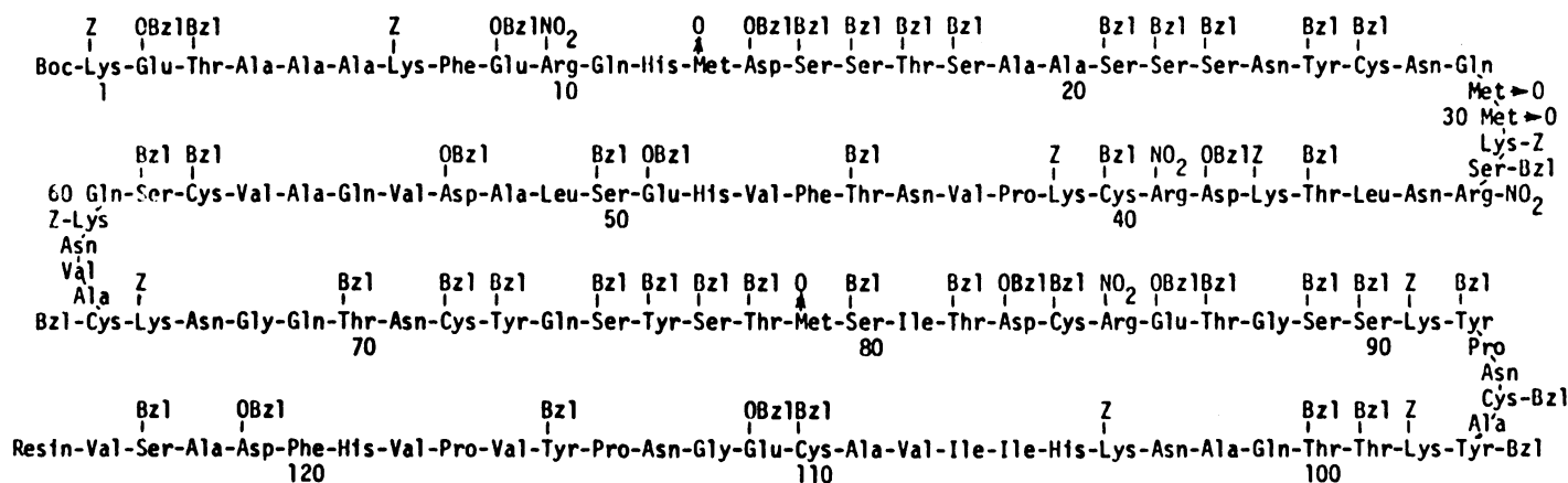
Fig. 10. Protected ribonuclease-resin.
