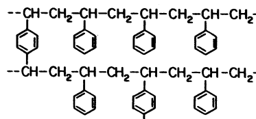
Fig. 3. Copoly(styrene-1%-divinylbenzene) resin.
