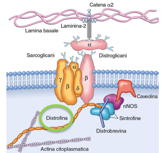
complesso distrofina-glicoproteine
