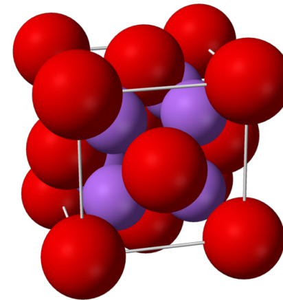
Na_2O
