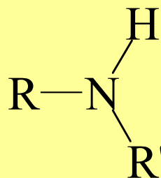
ammina secondaria
