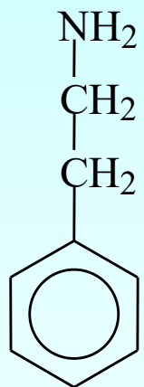
2-feniletanamina
