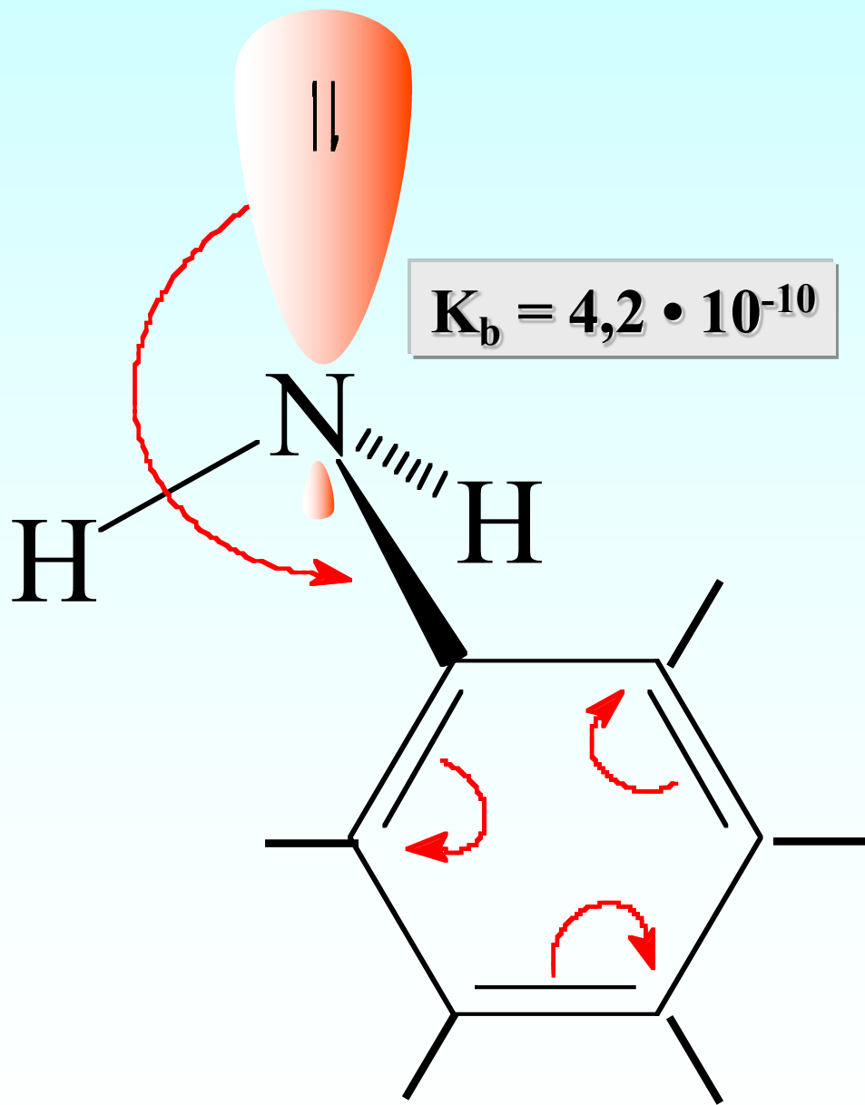
benzenammina
