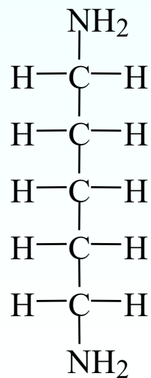
1,5-pentandiammina ( cadaverina )
