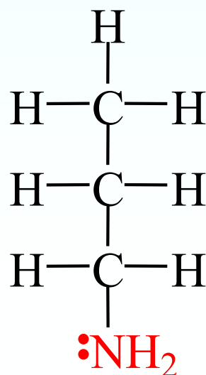
ammina primaria
