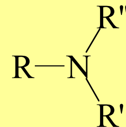
ammina terziaria
