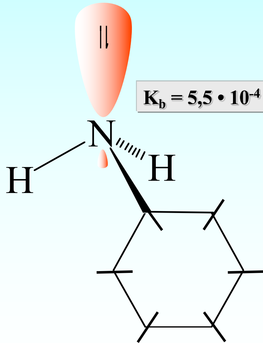
cicloesanammina
