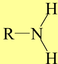
ammina primaria
