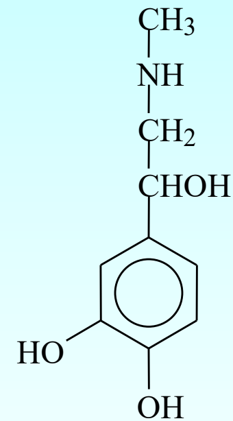
adrenalina
