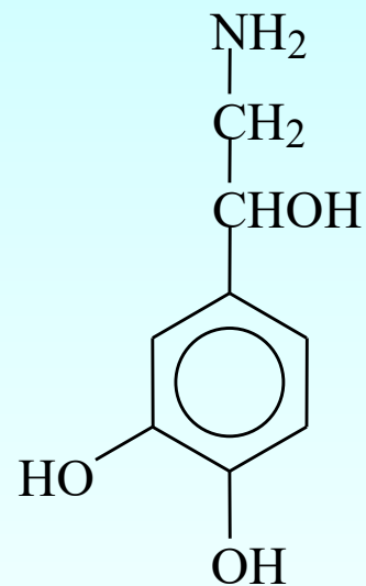
nor-adrenalina
