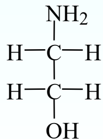
2-amminoetanolo ( etanolamina )
