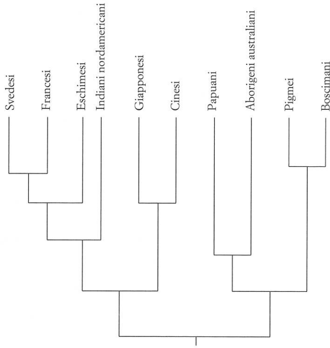
FIGURA 2 Albero filogenetico basato sui caratteri morfologici
