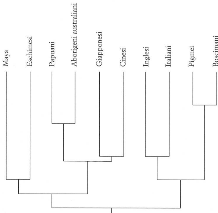
FIGURA I Albero filogenetico basato sui geni
