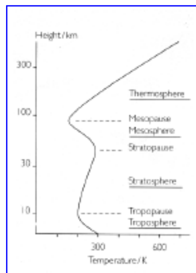
Fig. 1. Profilo della temperatura dell'atmosfera (Altezza/km - Termosfera - Mesopausa - Mesosfera - Stratopausa - Stratosfera - Tropopausa - Troposfera - Temperatura/K)
