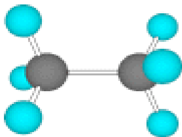
etano ( C_2H_6 )
