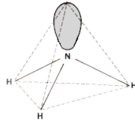
Ammoniaca NH_3
