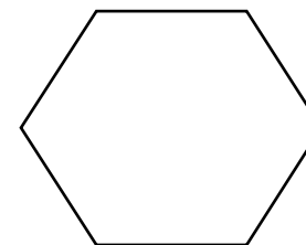
cicloesano
