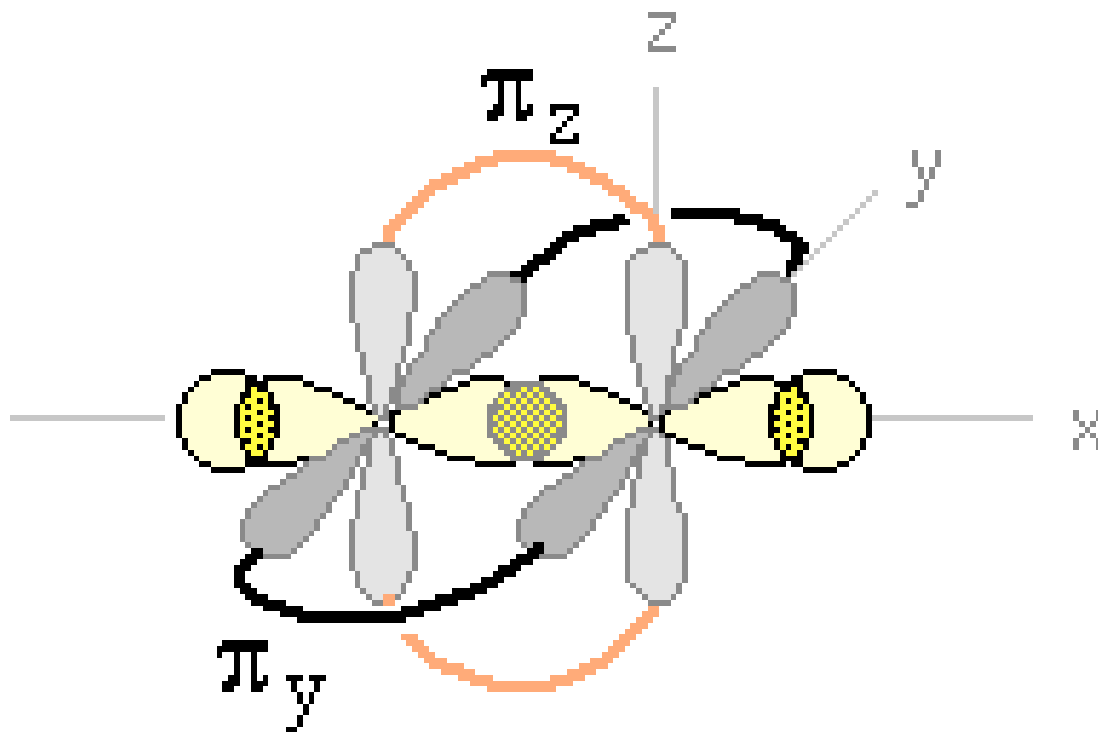
Etino: C_2H_2
