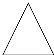
ciclopropano
