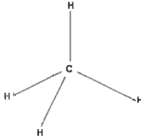
Metano: CH_4
