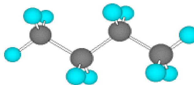
butano ( C_4H_{10} ).
