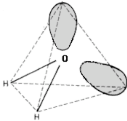
Acqua H_2O
