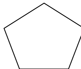
ciclopentano
