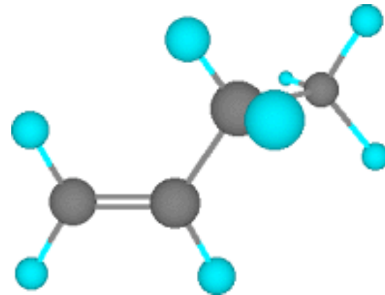
butene (C_4H_8) .
