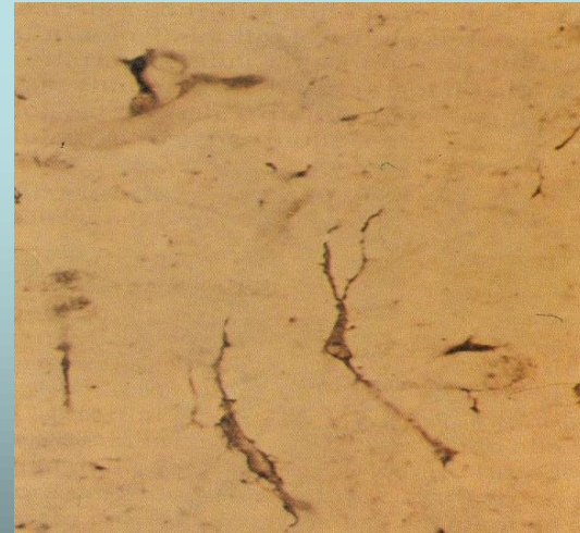
Microglia
