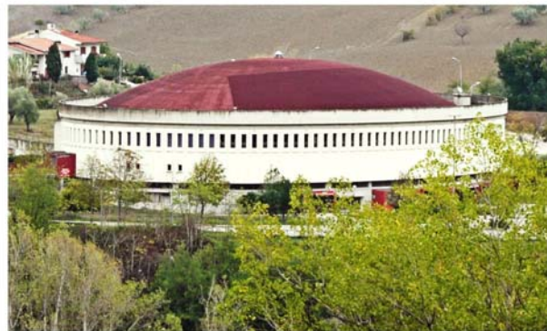
La più grande cupola a paraboloido ellittico in laterocemento mai realizzata nel mondo, costruita dall'ing. Giampiero Castellucci a Teramo nel 1980 per il PalaScapriano, il palazzetto dello sport. L'ellisse d'imposta del paraboloido ha assi di 63 metri e 45 metri.
