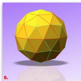
6. Completando tutta la "sfera" si ottengono Aste di due misure a seconda che si connettano a nodi su Vertici tipo A (5 Aste) o tipo B (a 6 Aste).
