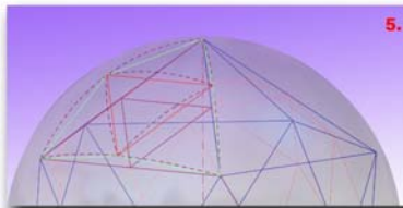
5. Supponiamo ora di voler realizzare una Cupola Geodetica sulla base dell'icosaedro. Per far ciò proiettiamo sulla sfera che circoscrive il poliedro i punti medi degli spigoli dell'icosaedro (operazione di Doubling), usando il centro della sfera come punto di proiezione. Si ottengono Triangoli equilateri BBB e Triangoli Isoscele ABB; e due tipi di Vertice A che coincide con il Vertici dell'Icosaedro e Vertice B.
