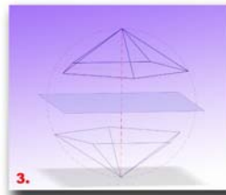
3. Costruisci ora una "calotta" dell'icosaedro, per simmetria costruiamo l'altra calotta. Per far ciò è necessario trovare l'asse dell'icosaedro costruendo la circonferenza che circoscrive il poliedro e riflettere la calotta al suo estremo. La posizione finale è ruotata di 36°
